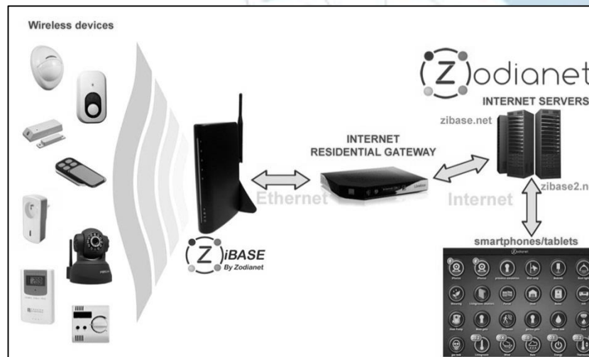
Struttura del sistema Zibase ( www.zodianet.com )
